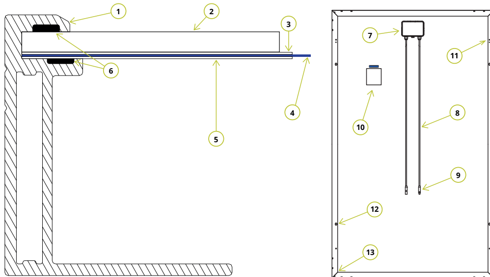
Rysunek 1 Przekrój panelu fotowoltaicznego i opis elementów
