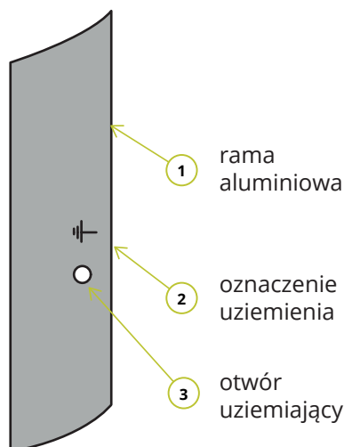
Rysunek 5 Otwór uziemiający
