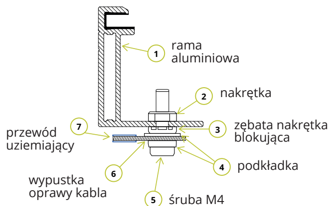
Rysunek 6 Sposób uziemienia panelu fotowoltaicznego
